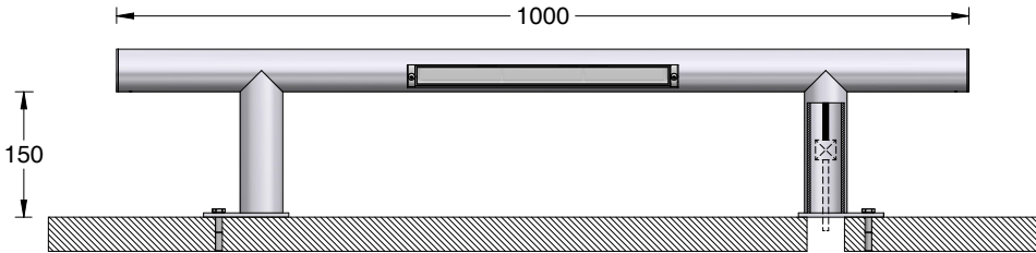
CHASSE-ROUE ROND
