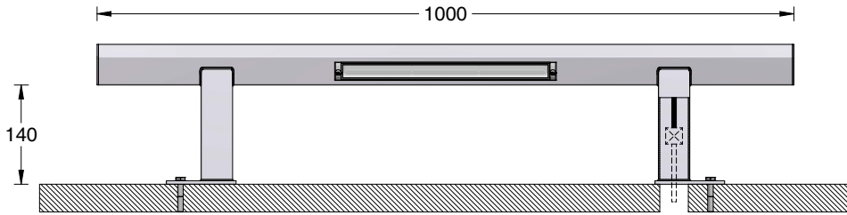
CHASSE-ROUE CARRÉ
